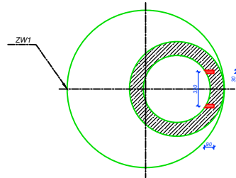
STUDZIENKA KANALIZACYJNA wg.DIN Ø1200 -rzut z góry
